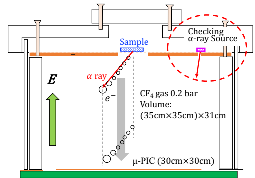
図4. 装置断面の概念図と較正線源の配置
