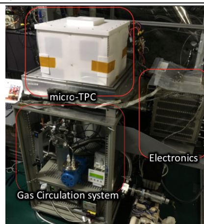
図1. 装置外観
